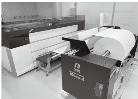
大径アンワインダー(送り出し装置)
